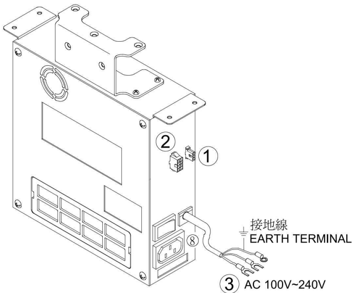
3 電源線 POWER LINE
