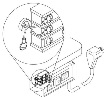
3 電源線 POWER LINE
